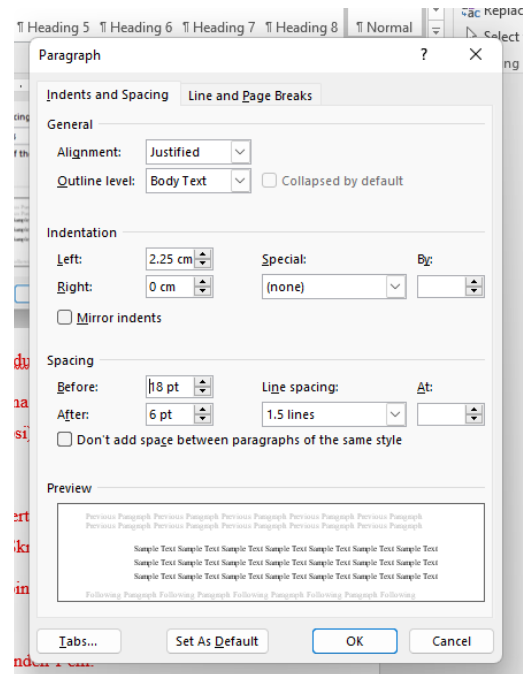
Gambar 4.2 Aturan Sub-bab
